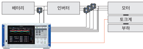
보정 테이블을 바탕으로 한 연산으로 토크계의 오차를 보정
